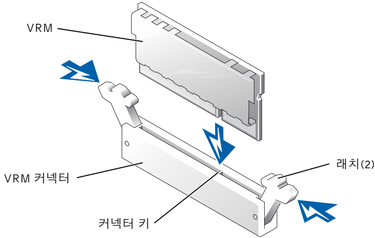
그림 6-2. VRM 설치
